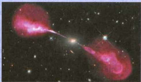
Рис. 187. Радиогалактика Геркулес А (3C 348)
