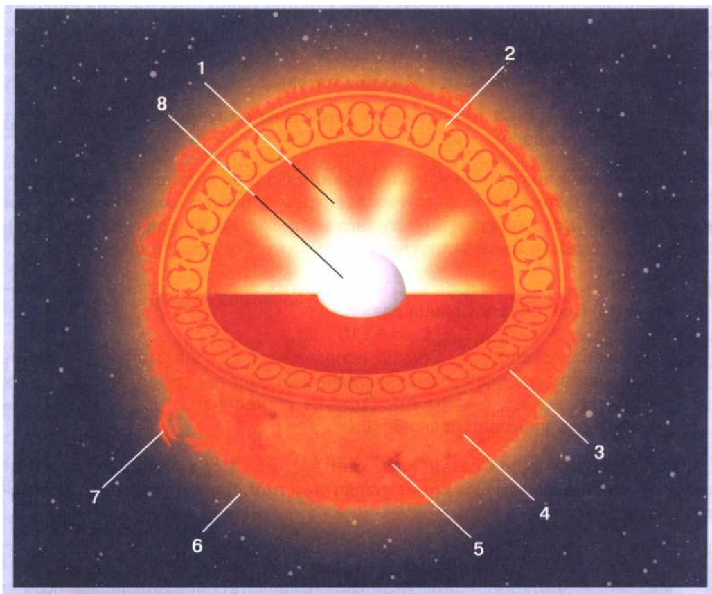
Рис. 138. Схема строения Солнца: 1 — зона лучистого переноса энергии; 2 — конвективная зона; 3 — хромосфера; 4 — фотосфера; 5 — солнечные пятна; 6 — корона; 7 — протуберанец; 8 — ядро
