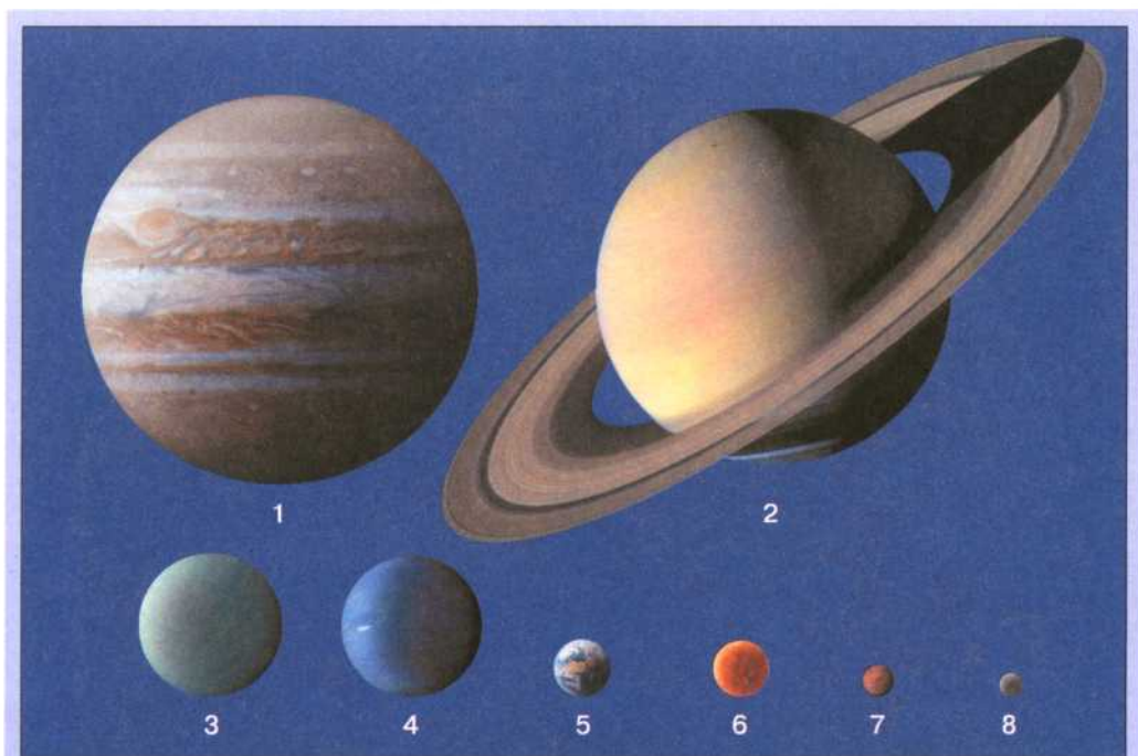
Рис. 78. Планеты Солнечной системы в едином масштабе: 1 — Юпитер; 2 — Сатурн; 3 — Уран; 4 — Нептун; 5 — Земля; 6 — Венера; 7 — Марс; 8 — Меркурий
