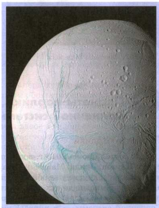
Рис. 101. Энцелад
