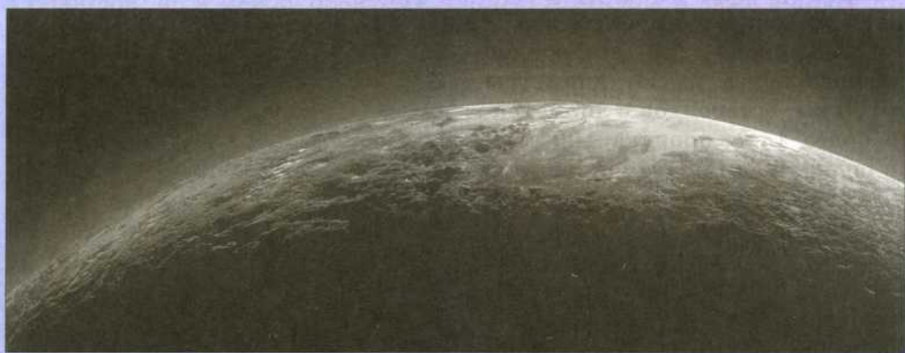
Рис. 105. Закат Солнца на Плутоне чётко выявляет наличие у него атмосферы, которая имеет сложную слоистую структуру. На снимке можно различить около 20 слоёв. Фото зонда «Новые горизонты» (New Horizons, NASA)
