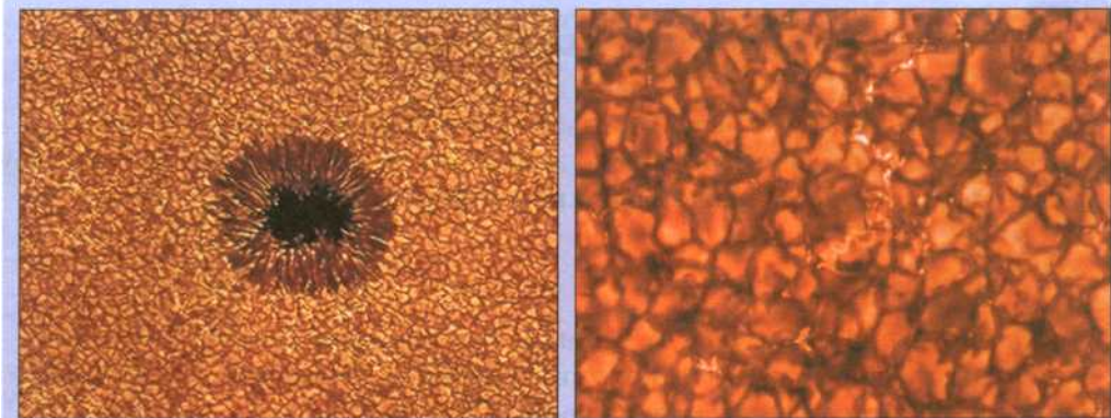
Рис. 139. Слева: грануляция солнечной фотосферы вокруг одиночного пятна. Справа: грануляция солнечной фотосферы (крупным планом). Размер одной гранулы составляет 700 км и более
