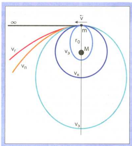
Рис. 73. Космические скорости
