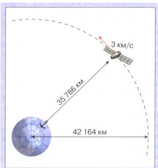
Рис. 75. Геостационарная орбита
