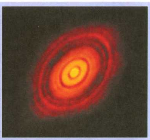
Рис. 176. Протопланетный диск
