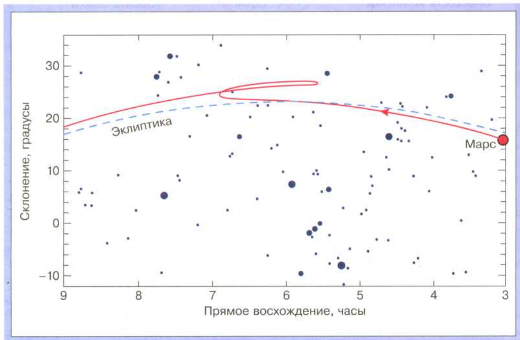
Рис. 55. Движение Марса по небу с июля 2007 г. по июнь 2008 г.
