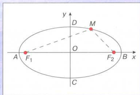
Рис. 68. Эллипс
