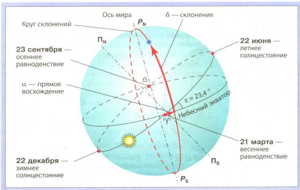
Рис. 49. За начало отсчёта прямого восхождения принята одна из двух точек пересечения небесного экватора с эклиптикой — точка весеннего равноденствия ( \gamma ). Линия P_N P_S — это ось эклиптики, параллельная оси земной орбиты
