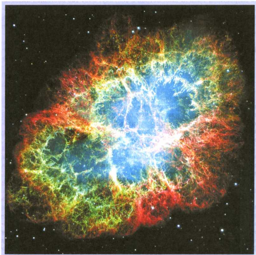
Рис. 158. Крабоподобная туманность (оптическое изображение). Голубой цвет (в центре) — синхротронное излучение, остальные цвета — излучение атомов различных газов
