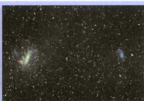
Рис. 179. Большое и Малое Магеллановы Облака
