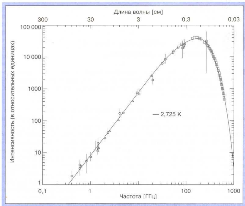
Рис. 192. Спектр фонового реликтового излучения. Различными значками показаны данные измерений (вертикальные отрезки — ошибки измерений). Сплошная линия — теоретическая кривая для спектра теплового излучения с T = 2,725 \text{ К}
