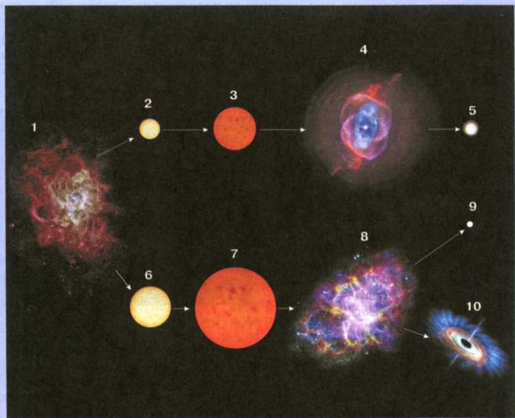
Рис. 156. Эволюция звёзд разной массы: 1 — газовой-пылевое облако; 2 — звезда солнечной массы; 3 — красный гигант; 4 — планетарная туманность; 5 — белый карлик; 6 — массивная звезда; 7 — красный сверхгигант; 8 — взрыв сверхновой; 9 — нейтронная звезда; 10 — чёрная дыра, окружённая аккреционным диском
