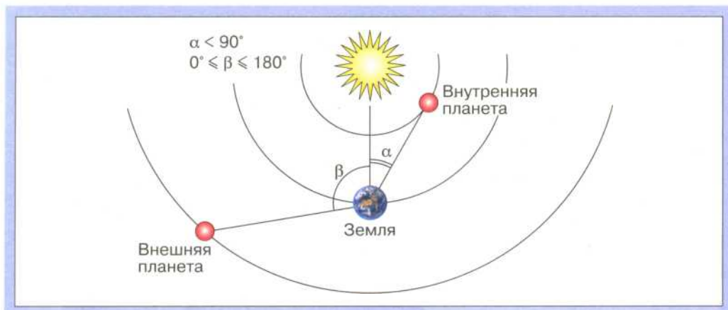
Рис. 58. Элонгация у внешних и внутренних планет
