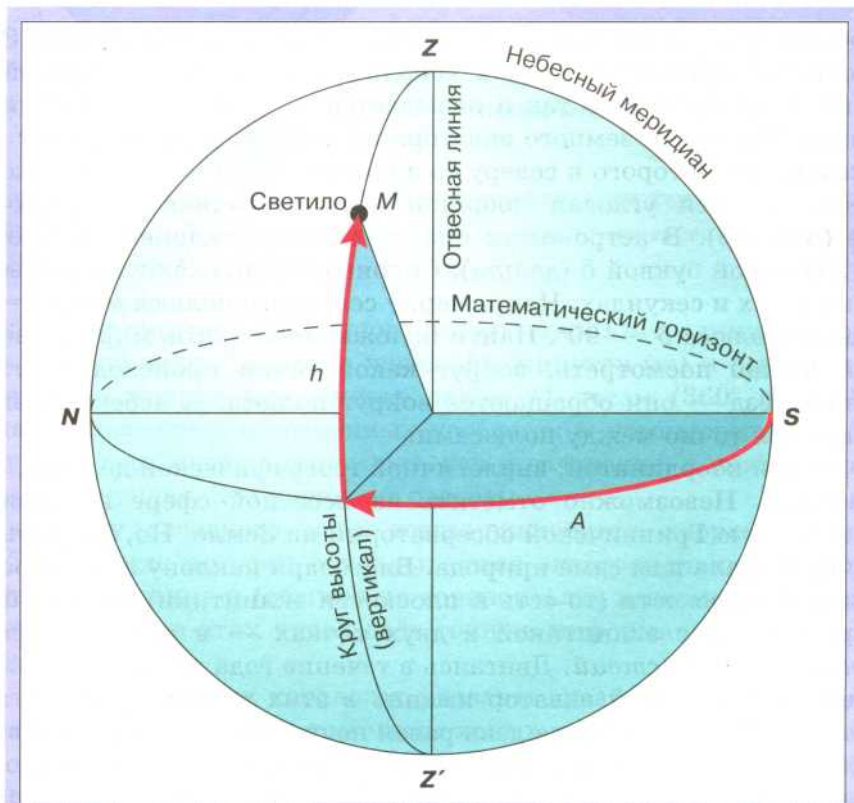
Рис. 47. Горизонтальная координатная система
