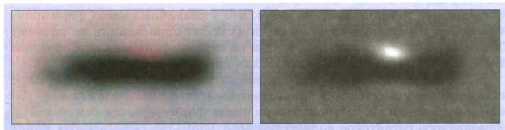
Рис. 175. Формирующиеся звёзды, окружённые непрозрачными газовой-пылевыми (протопланетными) дисками, в области Туманности Ориона
