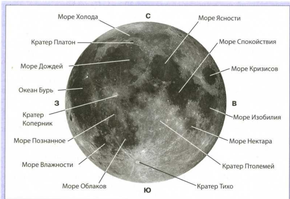
Рис. 81. Видимая с Земли сторона Луны
