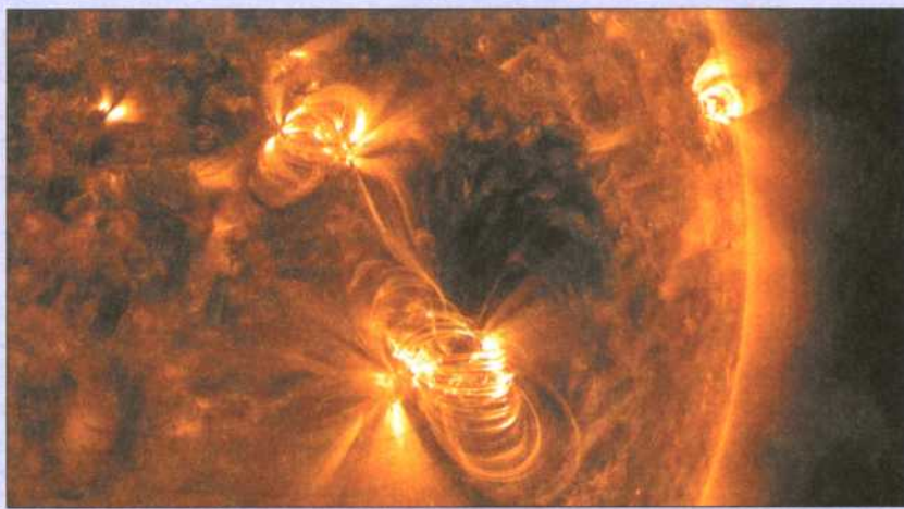
Рис. 144. Солнечные вспышки
