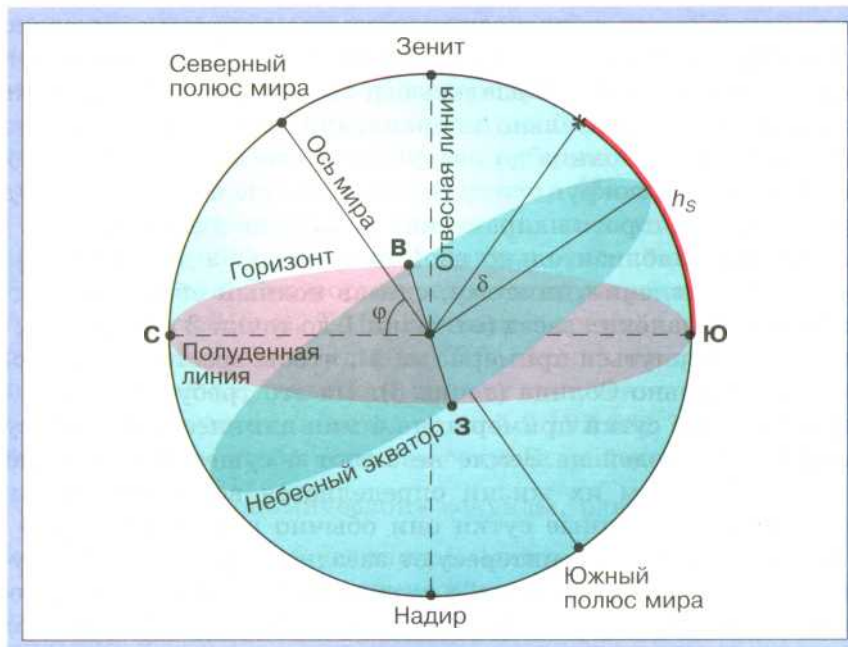
Рис. 52. Верхняя кульминация звезды с известным склонением ( \delta ) позволяет измерить географическую широту наблюдателя
