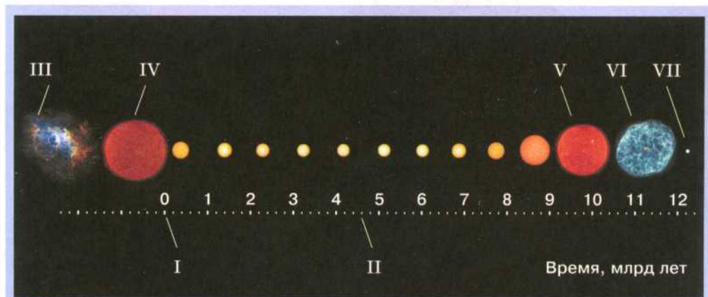
Рис. 150. Эволюция Солнца: I — начало термоядерной реакции; II — настоящее (4,57 млрд лет); III — часть молекулярного облака; IV — протозвезда; V — красный гигант; VI — планетарная туманность; VII — белый карлик
