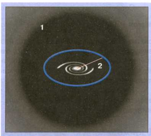
Рис. 184. Схема строения галактики.
