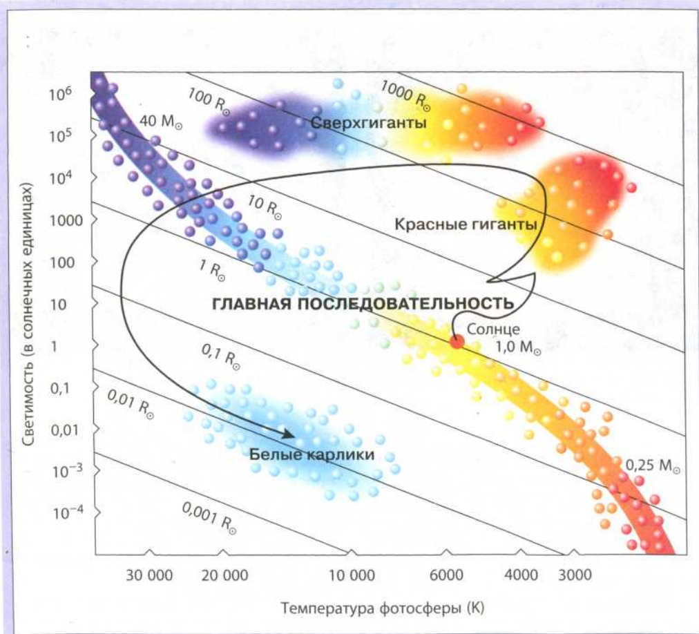
Рис. 153. Эволюционный трек звезды массой 1 M_{\odot}
