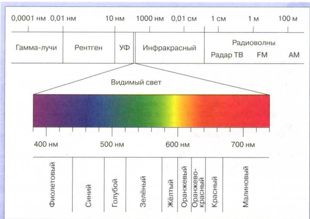
Рис. 130. Шкала электромагнитных волн. Область видимого света занимает узкую полоску между ультрафиолетовым и инфракрасным светом
